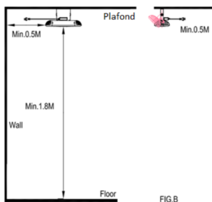
Montage plafond
