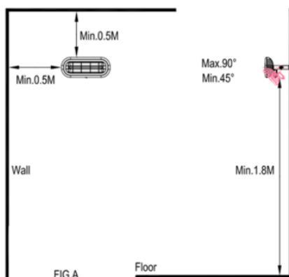
Montage Mural
